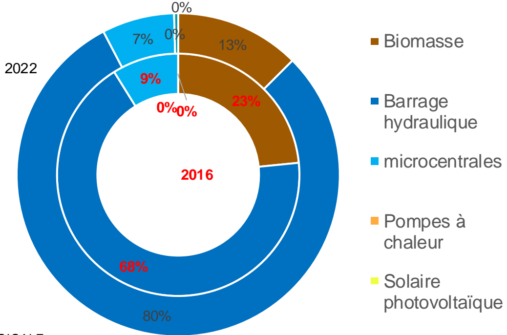
Comparaison de la répartition de production d'énergie par source entre 2016 et 2022
