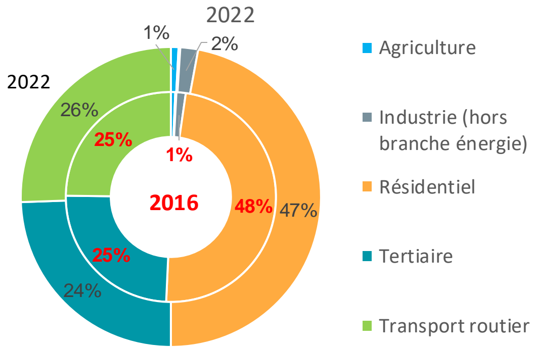
Comparaison répartition des consommations énergétiques par secteur d'activité entre 2016 et 2022
