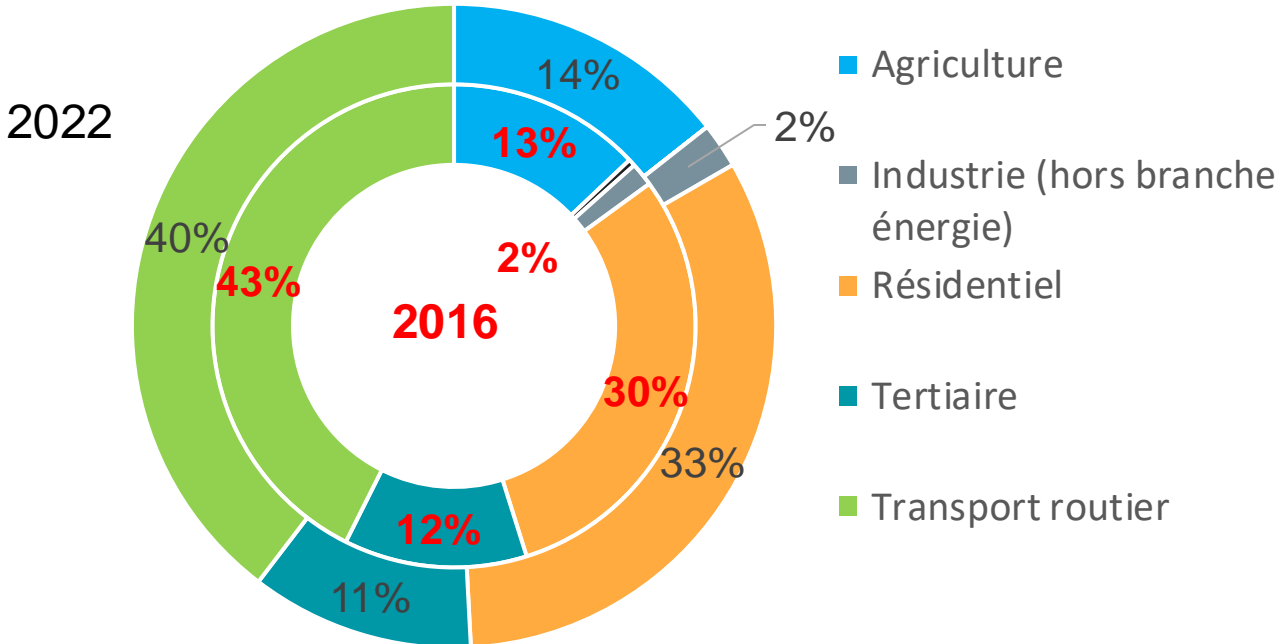
Comparaison de la répartition des émissions de gaz à effet de serre par secteur d'activité entre 2016 et 2022
