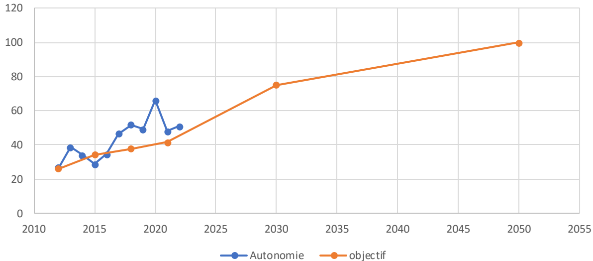
Autonomie énergétique par rapport aux objectifs du PCAET
