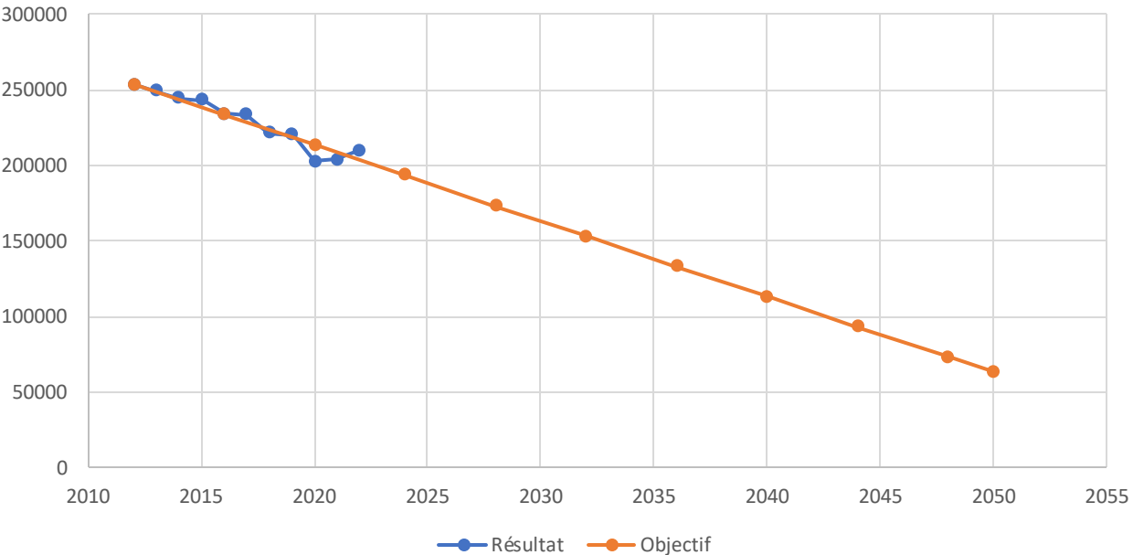
Evolution des émissions de gaz à effet de serre par rapport à l'objectif SRADDET (en teq CO2)
